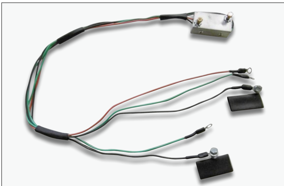
Kontaktgesteuerte Transistorzündanlage 110,00 €
